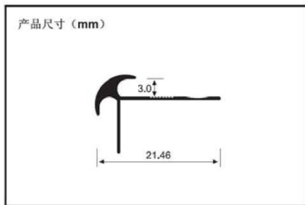
阳角收边
