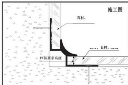
阴角收边
