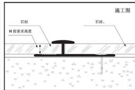
过度条
