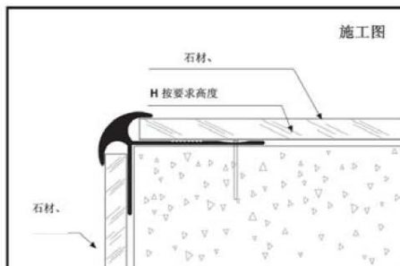
阳角收边
