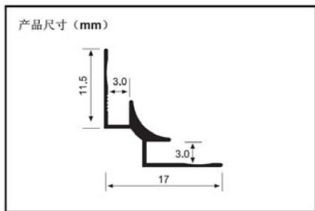
阴角收边
