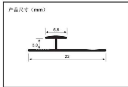
过度条
